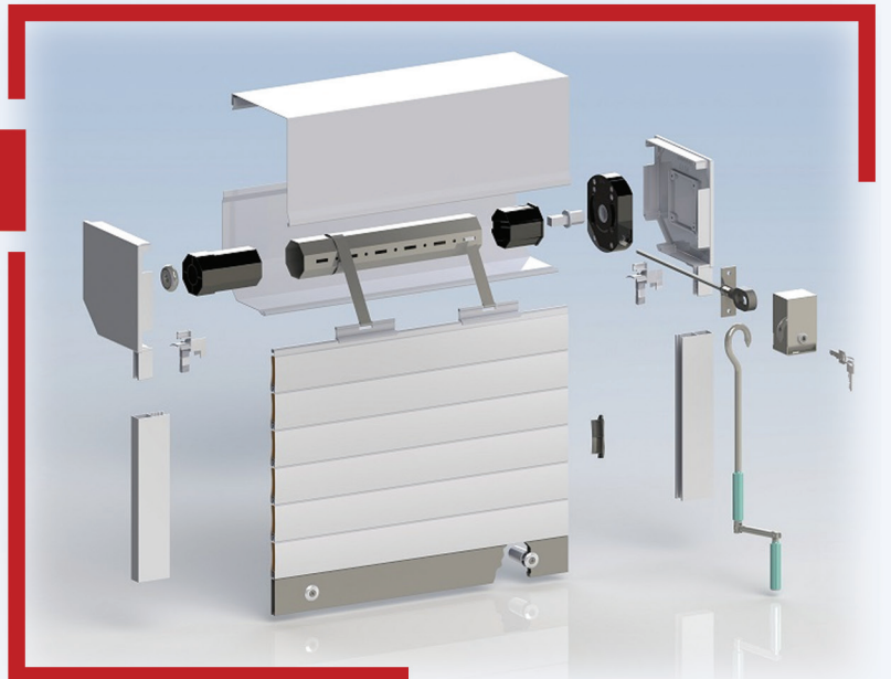
REDÜKTÖRLÜ PANJUR SİSTEMİ ROLLING SHUTTER SYSTEM WITH HANDLE
